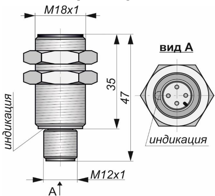
Габаритный чертеж
